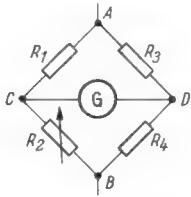
Bild 18.10. Wheatstone-Brücke zur Widerstandsmessung
