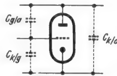
Bild 18.6. Röhrenkapazitäten bei der Triode
