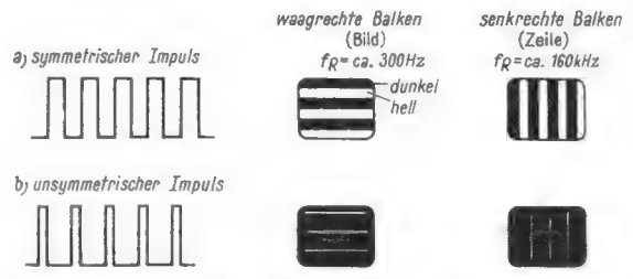
Bild 5. Rechteckimpulse und ihre Abbildung auf dem Bildschirm
