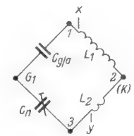
Bild 18.9. Umzeichnung von Bild 18.8 in eine Brückenschaltung
