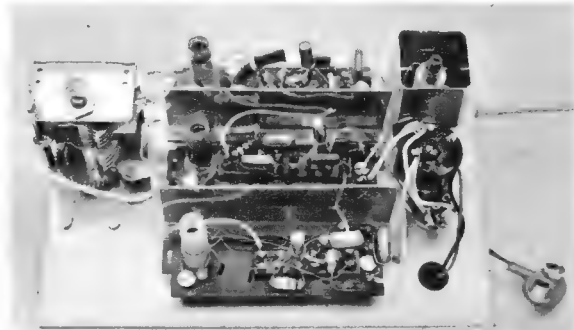
Bild 1. Ansicht des Mustergerätes. Die Stufen wurden als Bausteine ausgeführt und durch Zwischenbleche abgeschirmt
