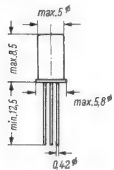
Bild 3. Abmessungen des Metallgehäuses der Transistoren
