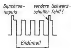
Bild 3. Bild- und Synchronsignal des hier beschriebenen Transistor-Balkengenerators
