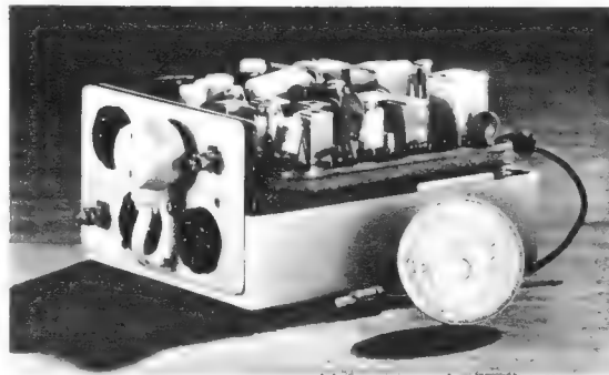
Bild 4. Der vollständige Zehnkanaal-Empfänger bestehend aus den Einheiten 195/2 und 195/4
