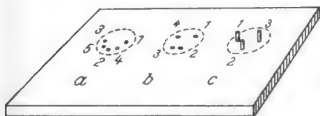
Arbeitsbrett für Lötarbeiten an Normsteckern und -Kupplungen
